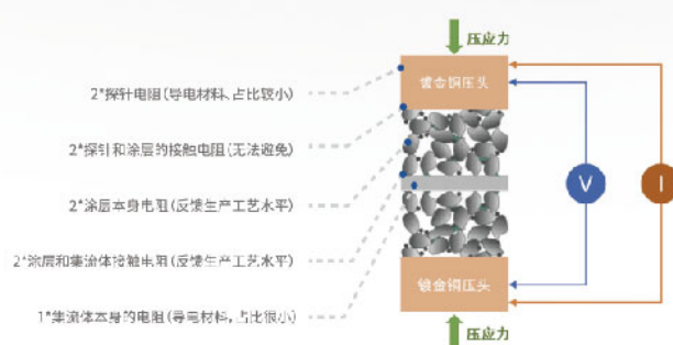
两探针测试原理
